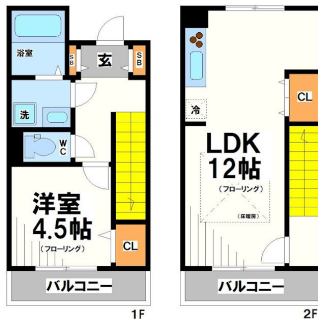
【間取り図】
