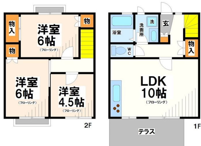
【間取り図】
