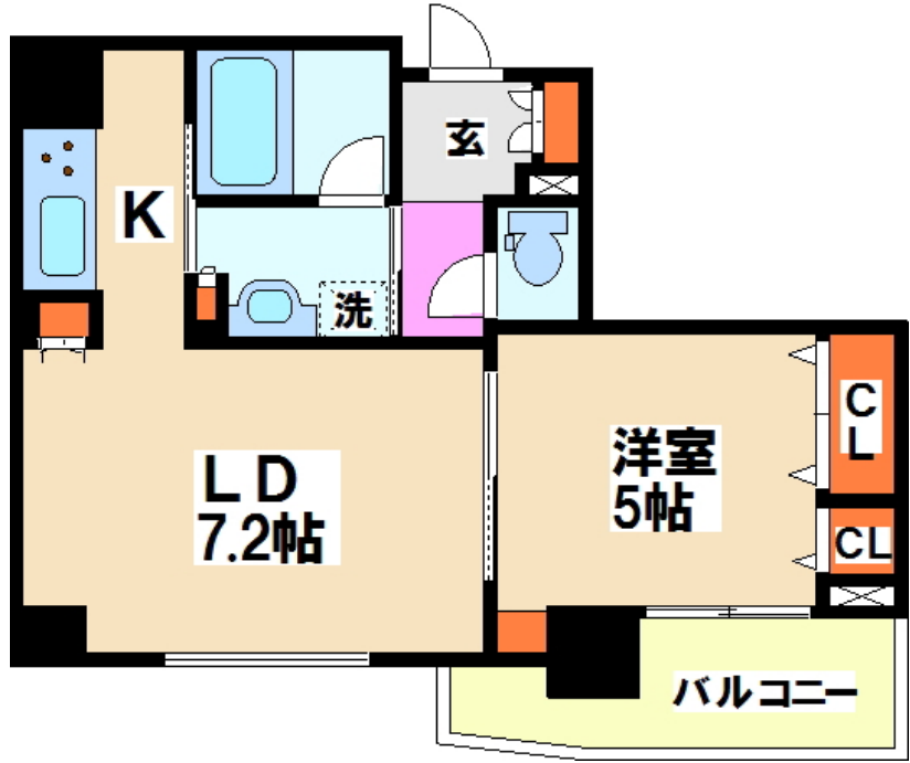
【間取り図】
