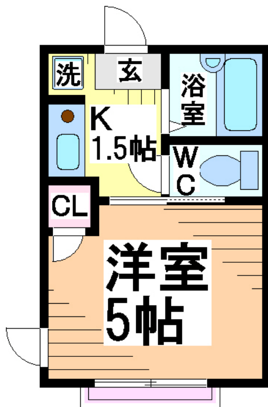
【間取り図】
