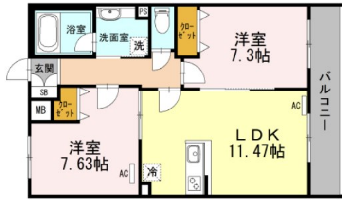
【間取り図】
